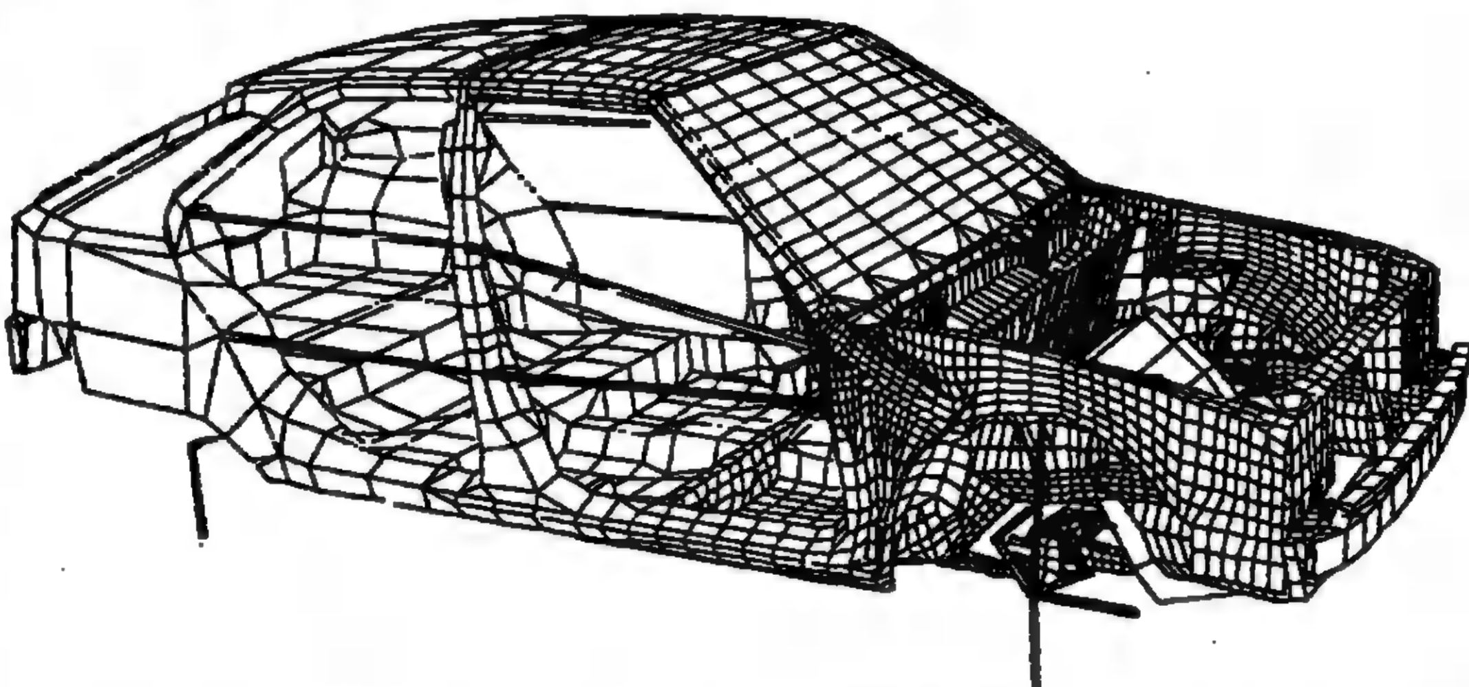
Le maillage d'une Citroën BX utilisé par le logiciel PAM-CRASH pour le calcul d'un choc.
